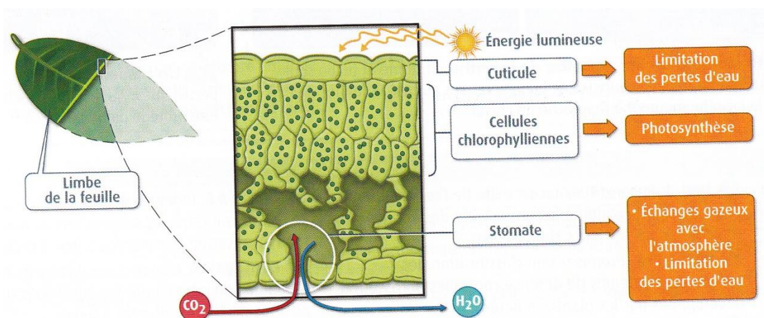
Les échanges entre une feuille et l'atmosphère.
